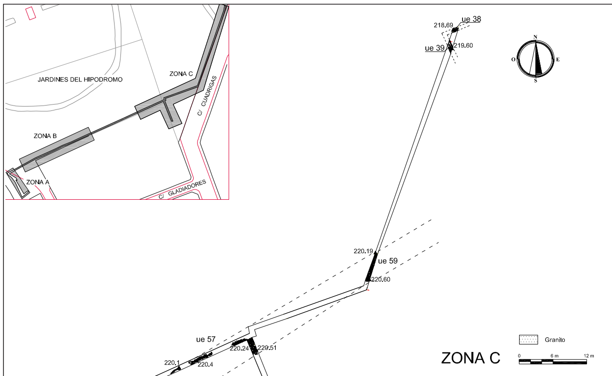
FIGURA 2 Planta general de la zona C.
